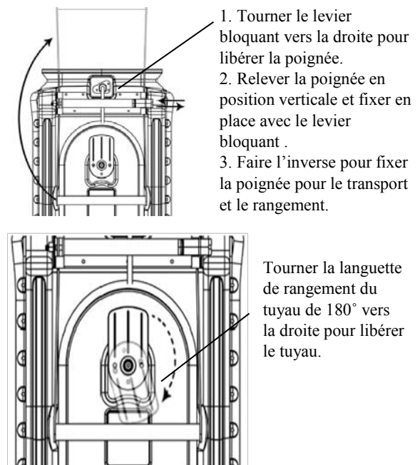
FIG. B : FIXATION DE LA POIGNÉE
