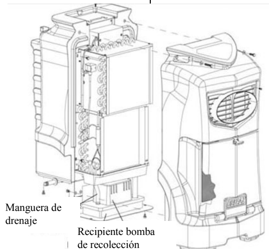
FIG. F: PANEL DE ACCESO A LA BOMBA
